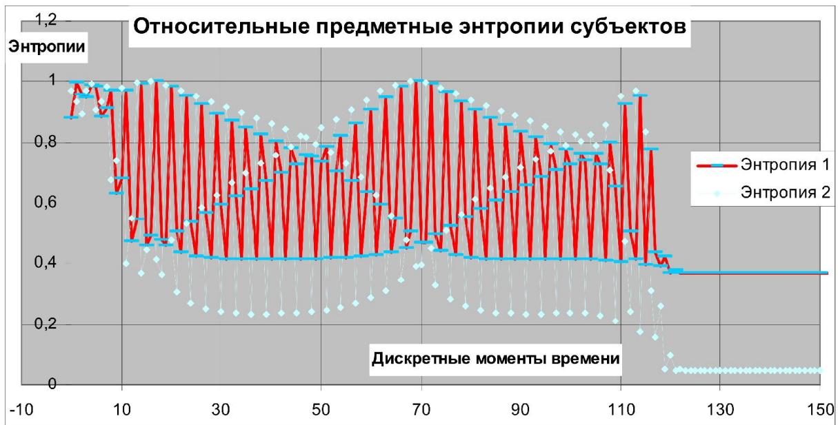
Рис. 5 – Динамика относительных предметных энтропий при двух субъектах и двух альтернативах
