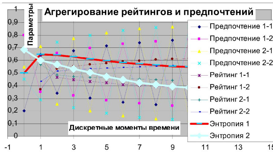
Рис. 2 – Параметры системы с двумя субъектами при наличии двух альтернатив
