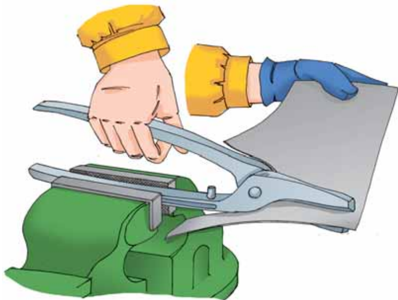
Мал. 75. Робота ножицями, закріпленими в лещатах
