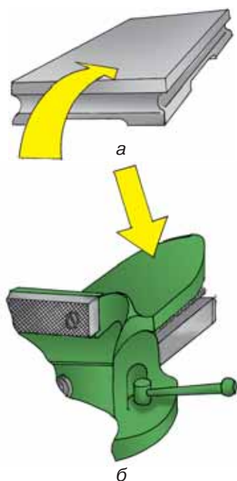
Мал. 56. Правильна плита (а) та ковадло слюсарних лещат (б)
