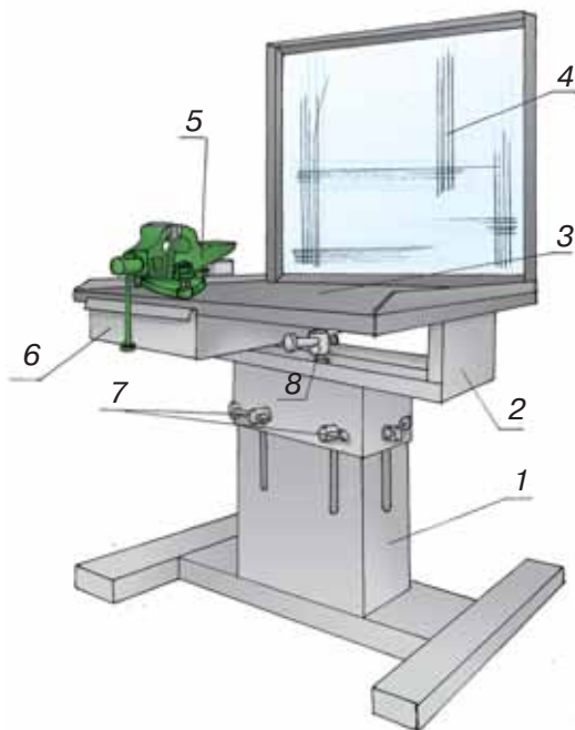
Мал. 8. Одномісний слюсарний верстак:
