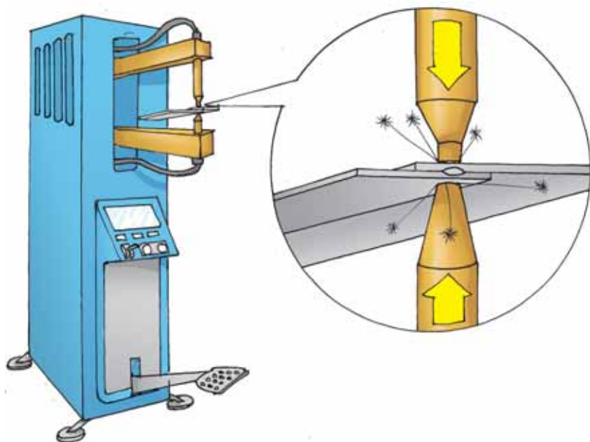
Мал. 106. Апарат для точкового зварювання тонколистового металу
