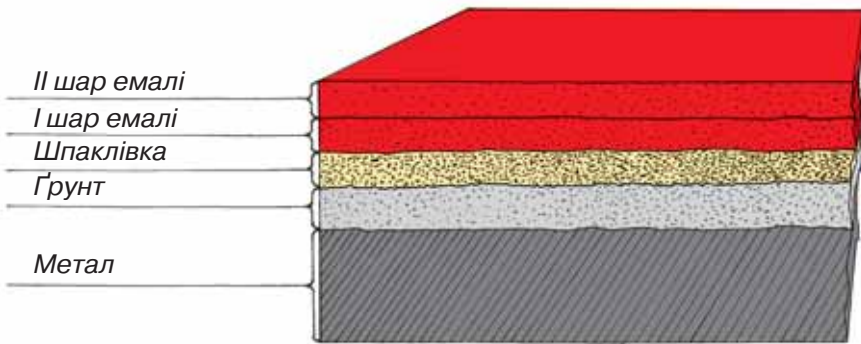
Мал. 146. Схема складних лакофарбових покриттів
