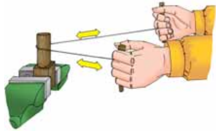
Мал. 119. Правлення дроту ковзанням навколо дерев'яного стержня
