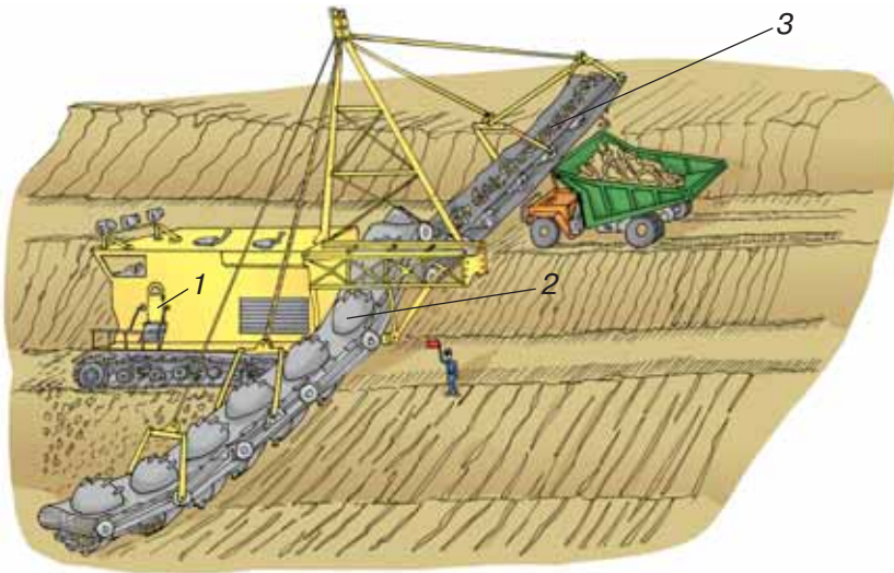
Мал. 3. Фрезерний екскаватор:
