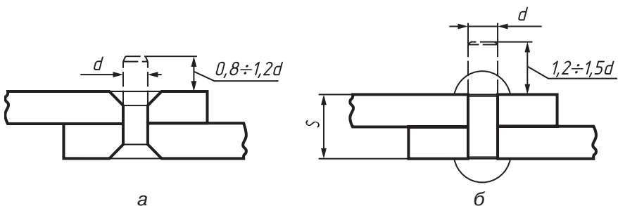
Мал. 113. Вибір довжини заклепки залежно від виду утвореної замикальної головки та товщини з'єднуваних деталей
