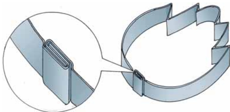
Мал. 100. Фальцовий шов
