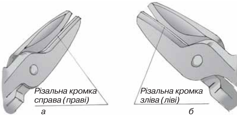
Рис. 73. Прямі ручні ножиці: а — праві; б — ліві
