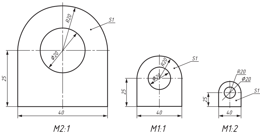
Мал. 47. Зображення деталі з тонколистового металу в різних масштабах та позначення на кресленнику товщини заготовки
