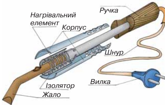
Мал. 104. Зовнішній вигляд та будова електропаяльника
