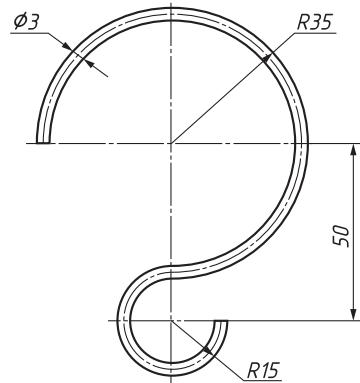
Мал. 125. Кресленик виробу із товстого дроту — гачка для вивішування наочності
