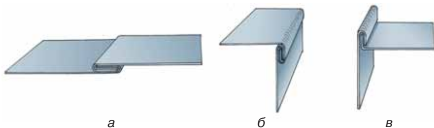
Мал. 107. Види фальцьових швів
