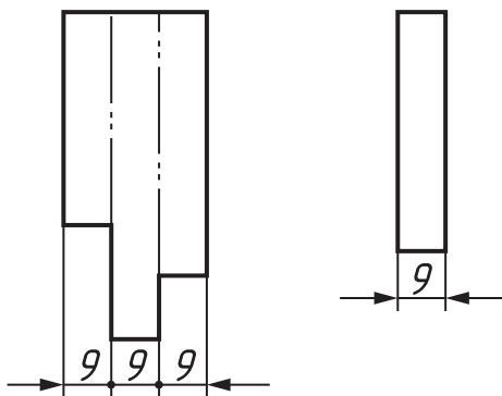
Мал. 55. Нанесення розмірів із застосуванням зустрічних стрілок
