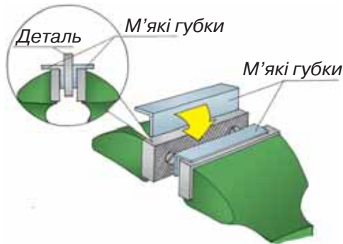
Мал. 96. М'які накладки на губки лещат
