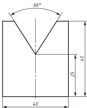
Мал. 48. Нанесення лінійних та кутових розмірів на кресленнику
