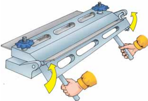
Мал. 98. Пристаювання для гнуття тонколистового металу на заданий кут
