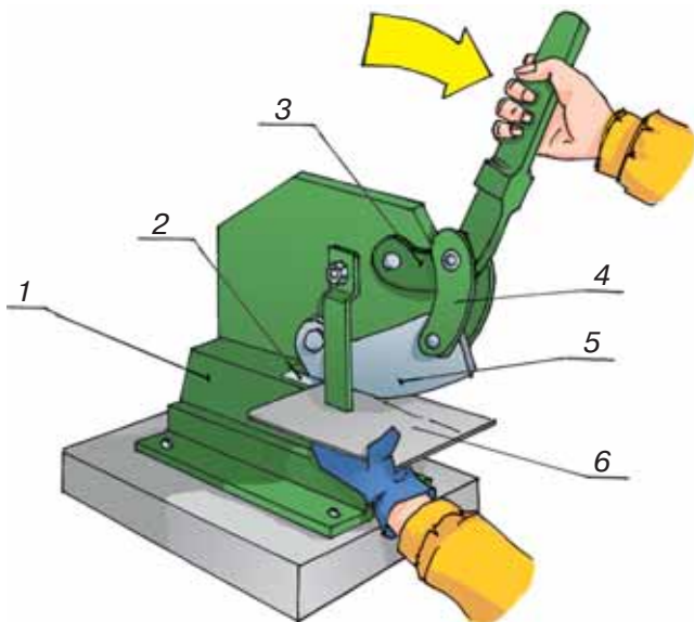
Мал 78. Різання металу на ручних важільних ножицях
