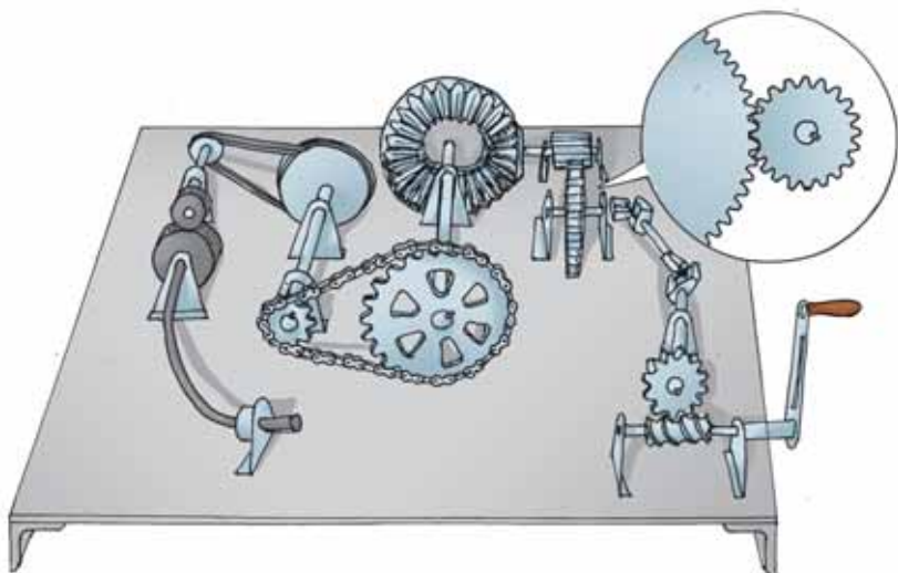
Мал. 162. Модель різних видів передач
