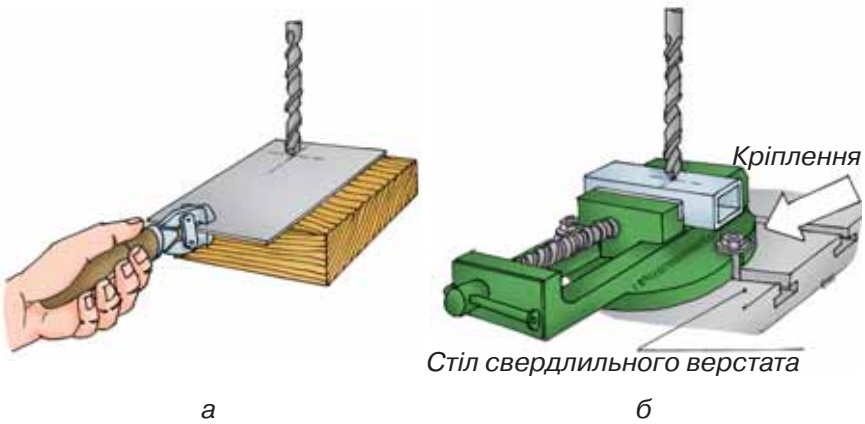
Мал. 174. Закріплення заготовки під час свердлення: а — у ручних лещатах; б — у машинних лещатах
