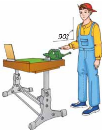
Мал. 11. Перевірка правильності вибору висоти слюсарного верстака
