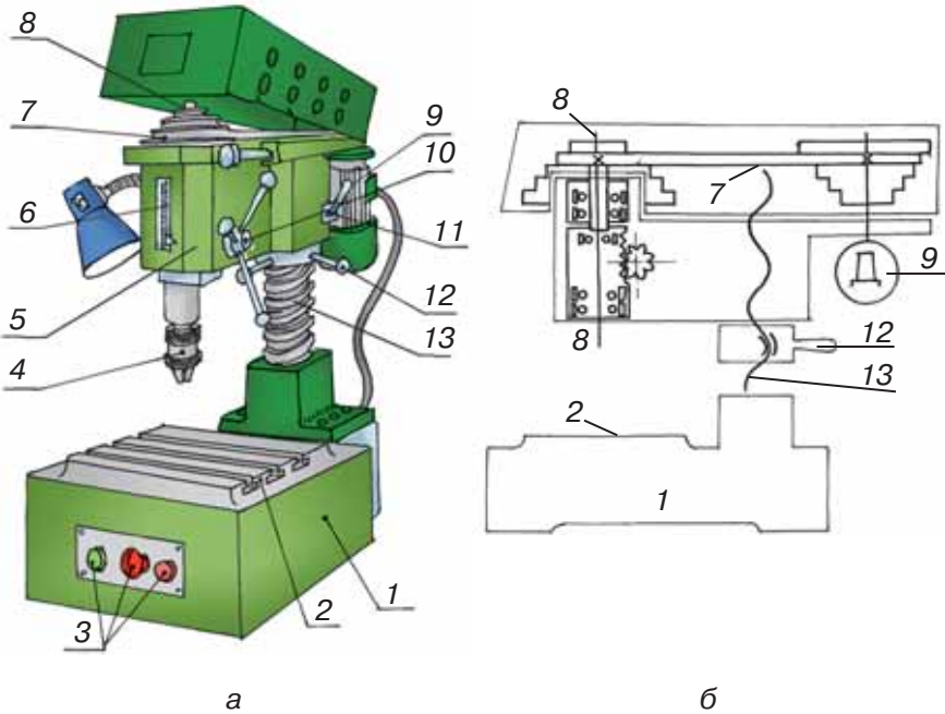
Мал. 172. Настільний свердлильний верстат 2М112: а — будова; б — кінематична схема; 1 — станина (плита); 2 — стіл; 3 — кнопки «Пуск», «Стоп», «Реверс»; 4 — патрон; 5 — бабка шпинделя; 6 — шкала; 7 — клиновий пас; 8 — шпindelь; 9 — електродвигун; 10 — штурвал; 11, 12 — рукоятки кріплення; 13 — гвинт-колона
