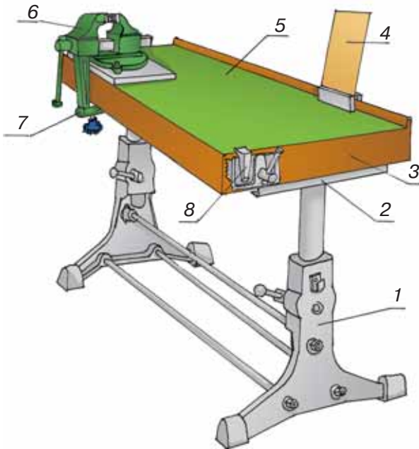
Мал. 7. Універсальний стіл-верстак:
