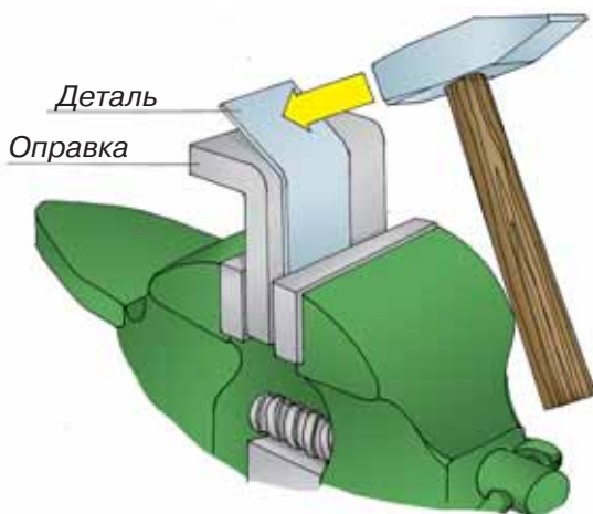
Мал. 95. Гнуття заготовки в лещатах по оправці
