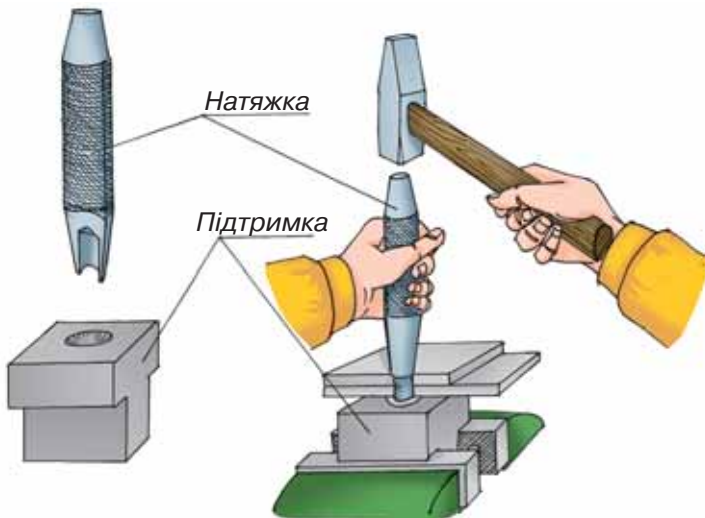
Мал. 115. Застосування натяжки та підтримки
