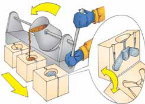
Мал. 20. Розливання рідкого металу
