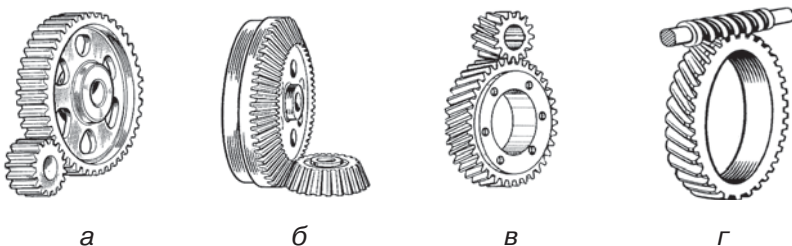
Мал. 164. Основні типи зубчатих передач:
