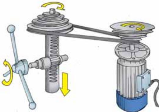
Мал. 172. Настільний свердлильний верстат 2М112: а — будова; б — кінематична схема; 1 — станина (плита); 2 — стіл; 3 — кнопки «Пуск», «Стоп», «Реверс»; 4 — патрон; 5 — бабка шпинделя; 6 — шкала; 7 — клиновий пас; 8 — шпindelь; 9 — електродвигун; 10 — штурвал; 11, 12 — рукоятки кріплення; 13 — гвинт-колона
