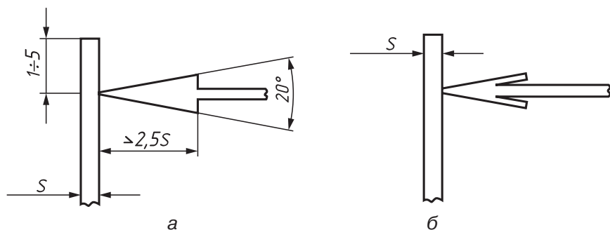
Мал. 49. Вимоги до накреслення розмірної стрілки
