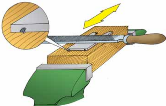
Мал. 143. Зачищення деталі напилком
