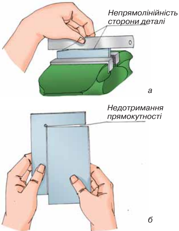
Мал. 88. Контроль обробленої поверхні за допомогою лінійки (а) та кутника (б)
