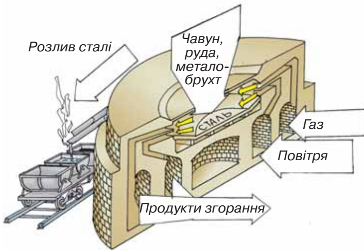
Мал. 22. Мартенівська піч та її внутрішня будова
