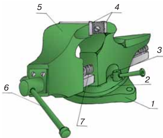
Мал. 10. Будова поворотних слюсарних лещат:
