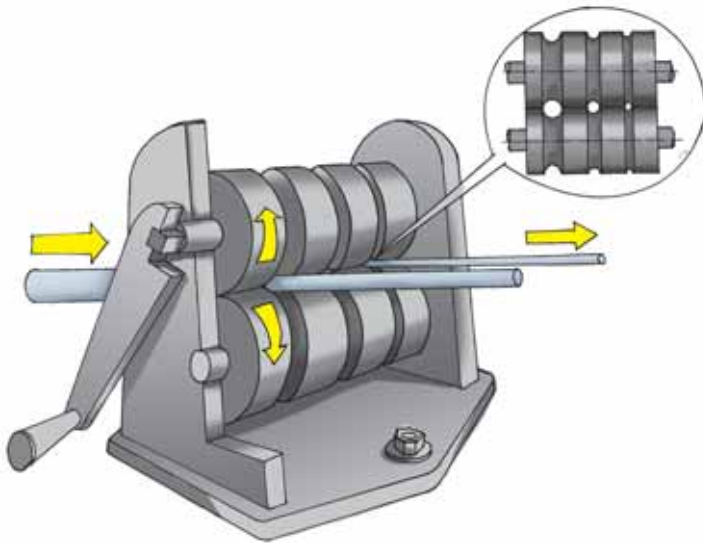
Мал. 25. Прокатування дроту
