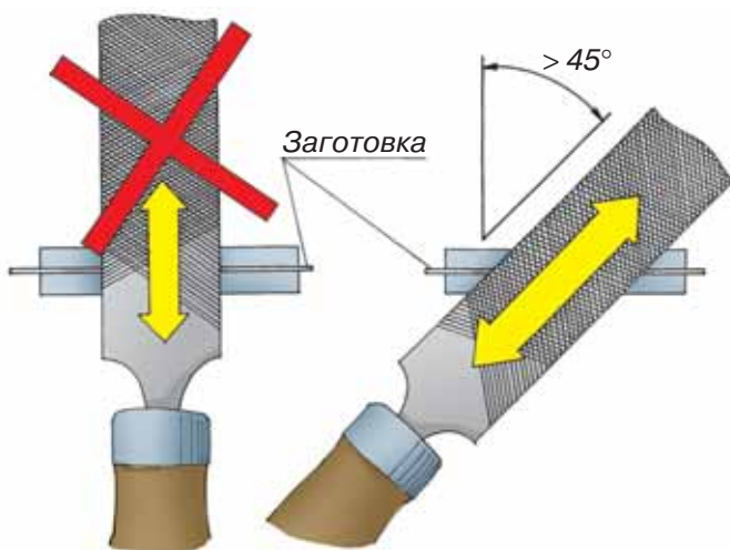
Мал. 89. Повздовжнє обпилювання тонкої заготовки
