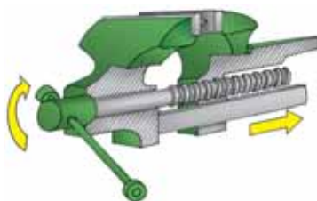
Мал. 167. Гвинтова передача
