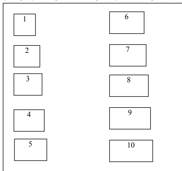
Рис. 3. набір прямокутників із різним співвідношенням сторін.
