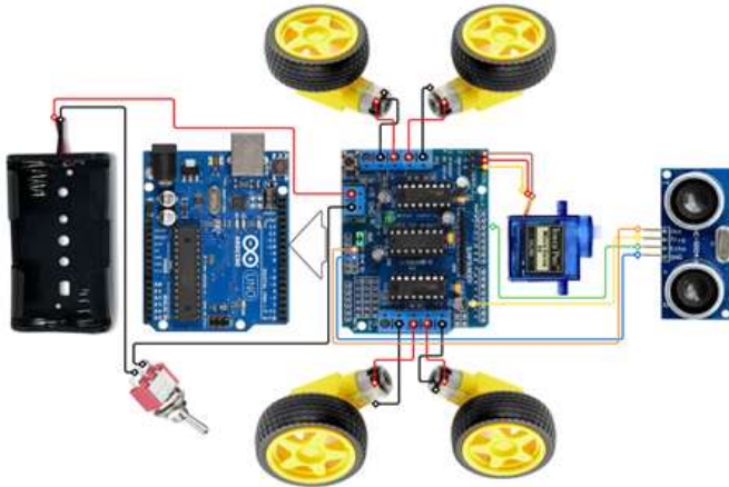
Рис. 2 Схема з'єднання компонентів мобільного робота
