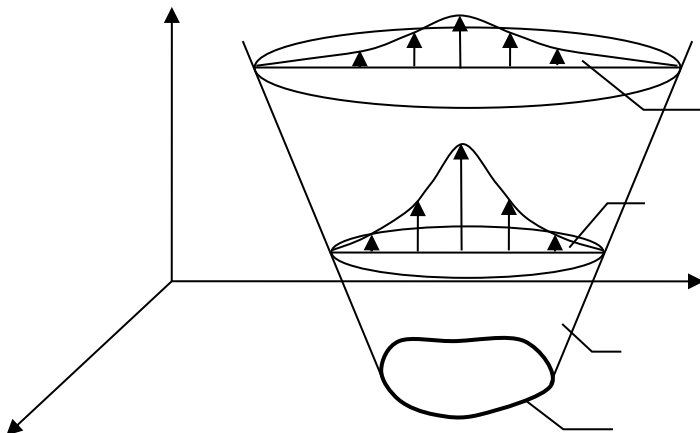
Рис. 1. Висхідний потік на розливом рідини, що горить: 1 – розлив горючої рідини; 2 – висхідний потік над осередком горіння; 3 – розподіл швидкостей у потоці на висоті z_1 ; 4 – розподіл швидкостей у потоці на висоті z_2 > z_1
