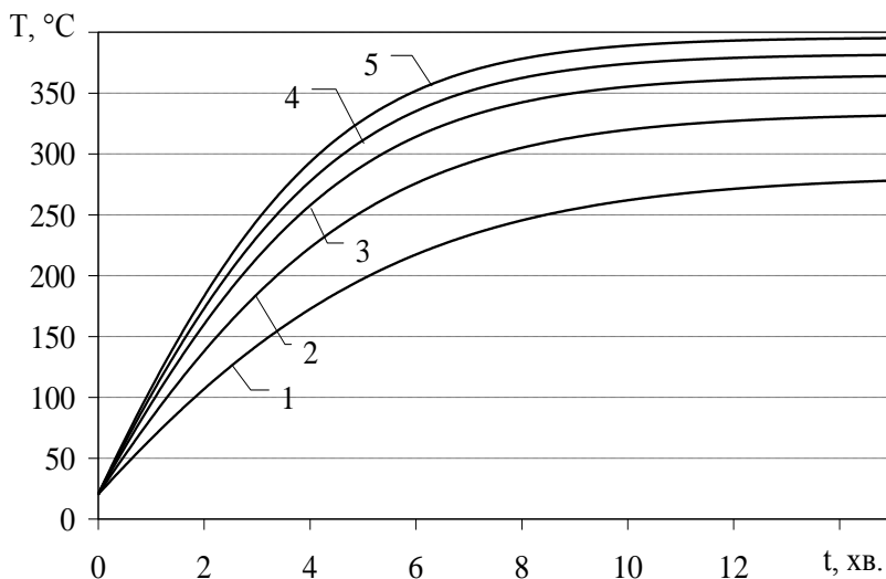
Рис. 1. Динаміка зміни температури зовнішньої поверхні покрівлі резервуара з боку пожежі при різних швидкостях вітру: 1 – w=0 ; 2 – w=1 м/с; 3 – w=2 м/с; 4 – w=3 м/с; 5 – w=5 м/с
