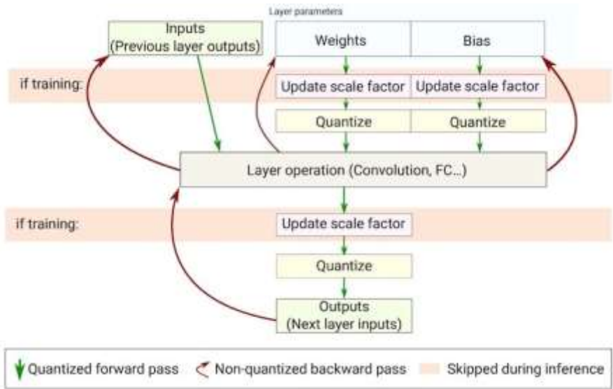
Рисунок 3 – процес квантування під час навчання.
