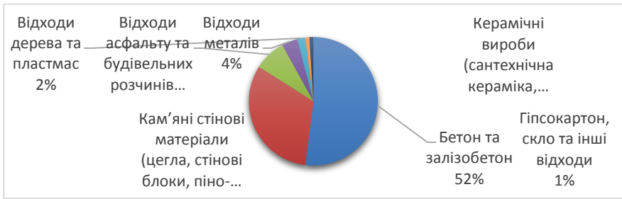
Рис. 1 Склад будівельних відходів за масовим вмістом
