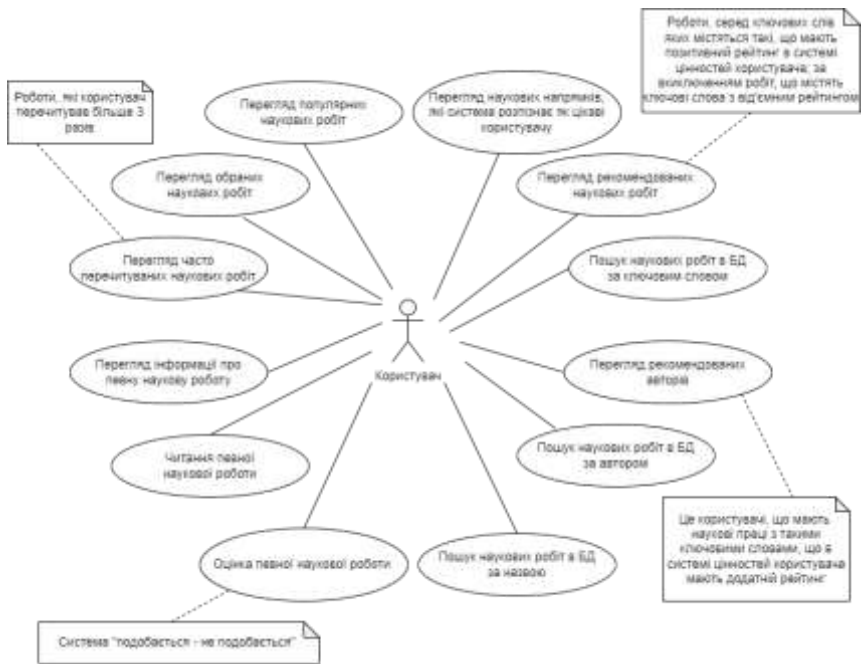
Рисунок 1. UML-діаграма прецедентів системи формування адаптивного веб-інтерфейсу користувача
