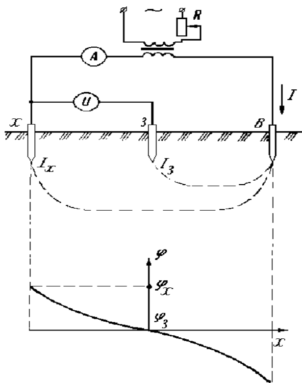
Рис. Б.1.3. Вимірювання опору захисного заземлення методом амперметра і вольтметра
