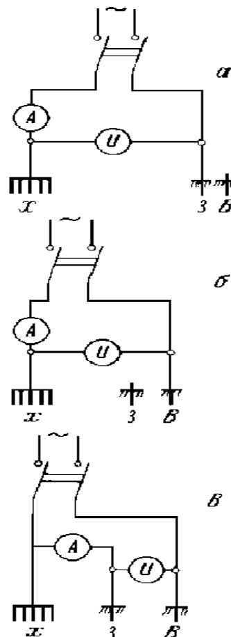
Рис.Б.1.4. Вимірювання опору заземлення методом трьох вимірювань
