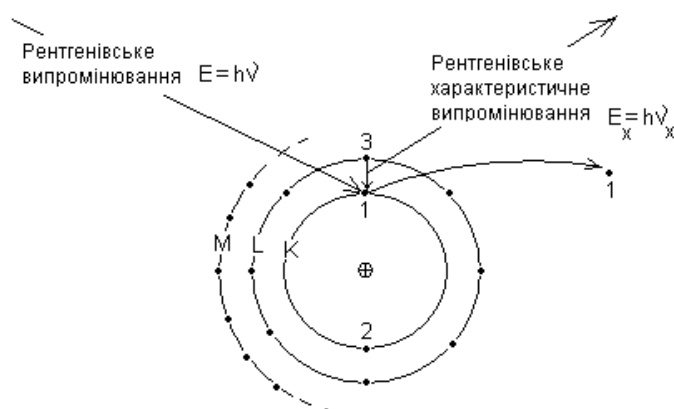
Рис.4.2. Виникнення рентгенівського характеристичного випромінювання K\alpha лінії в результаті флуоресценції.
