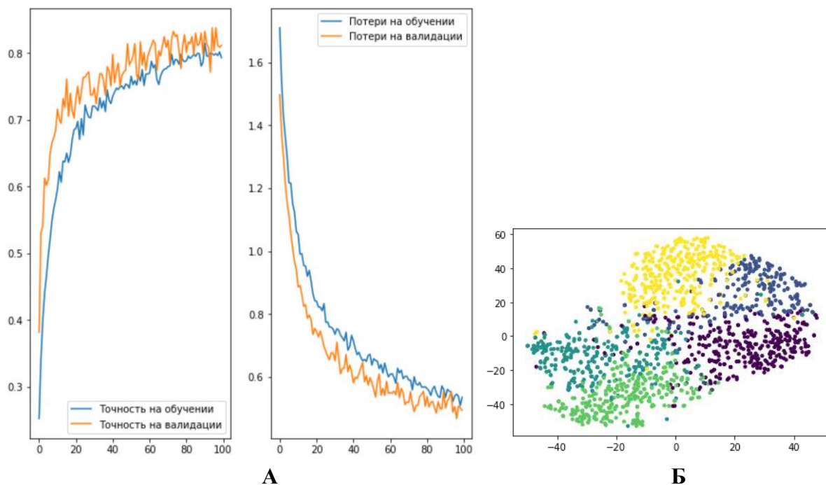
Рисунок 4 – результати навчання моделі (а) і вектора ознак на передостанньому шарі (б) моделі на базі EfficientNetB2
