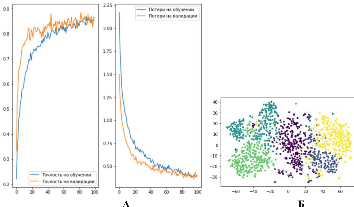
Рисунок 5 – результати навчання моделі (а) вектора ознак на передостанньому шарі (б) моделі на базі MobileNetV3Large
