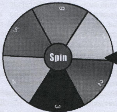
Рис. 1. Генератор чисел
