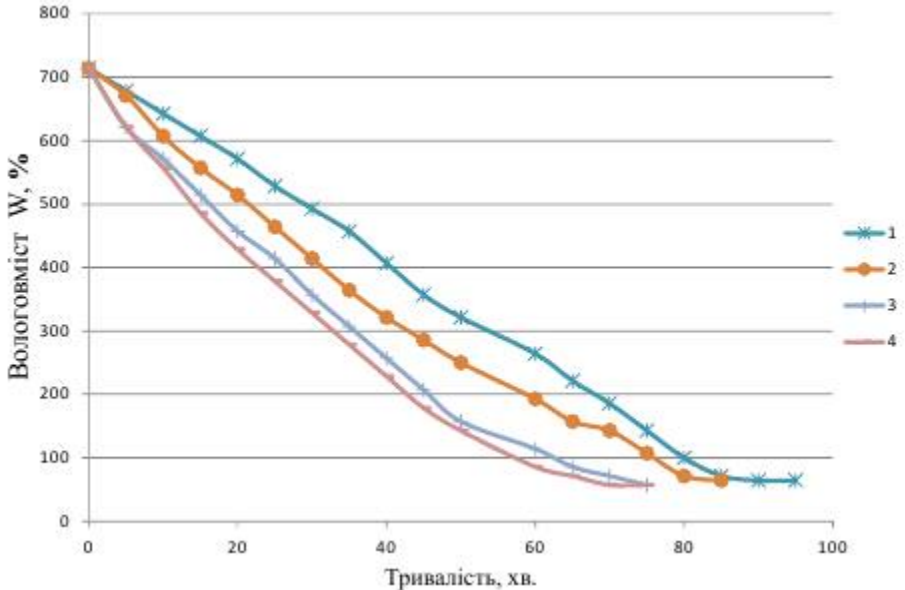
Рис. 1 - Криві комбінованого сушіння буряка при температурах, °С: 1 - 50, 2 – 60, 3 – 70, 4 – 80.
