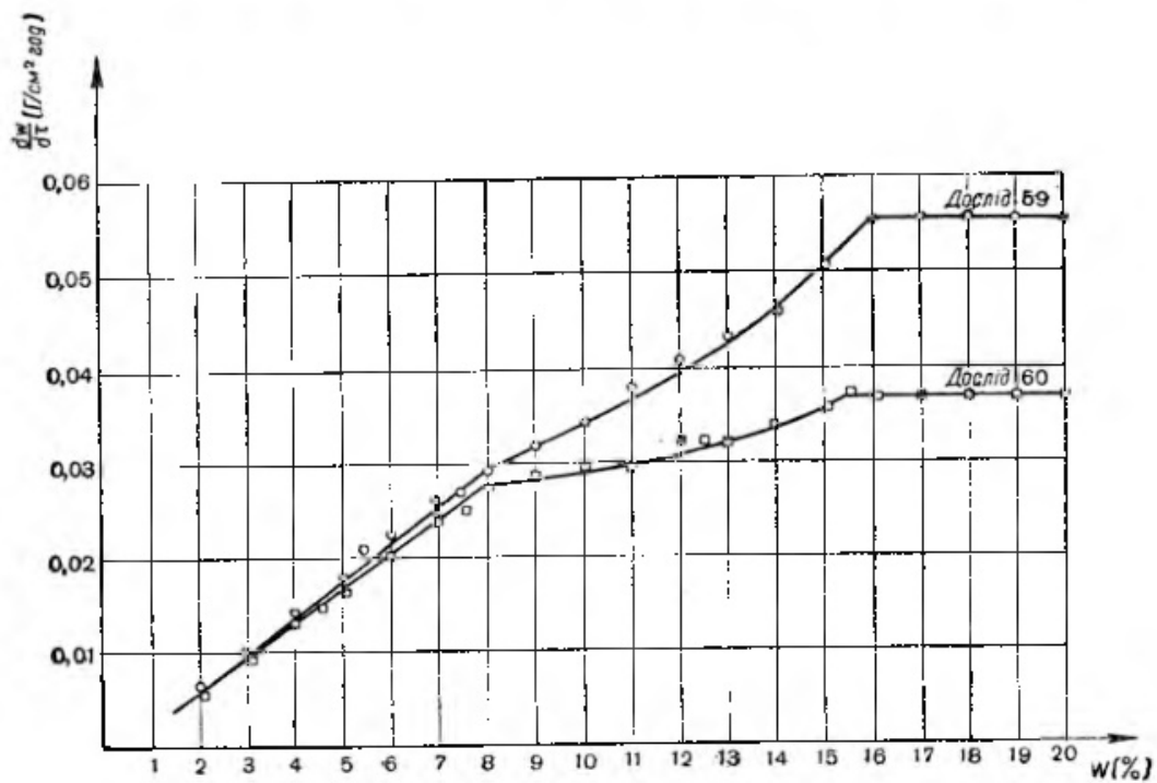
Рис. 9. Криві швидкості сушіння Часоварської II глини.
