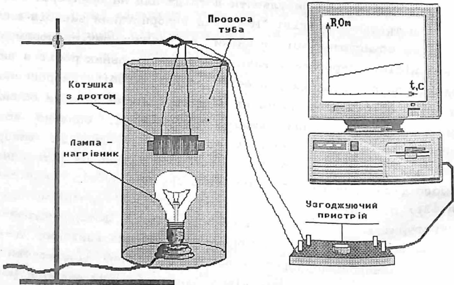
Мал. 3. Установка для дослідження зміни опору провідника при нагріванні
