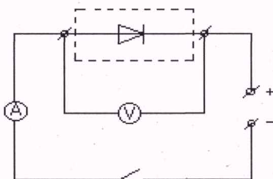
Рис. 2. Зміна полярності вмикання “чорної скриньки”
